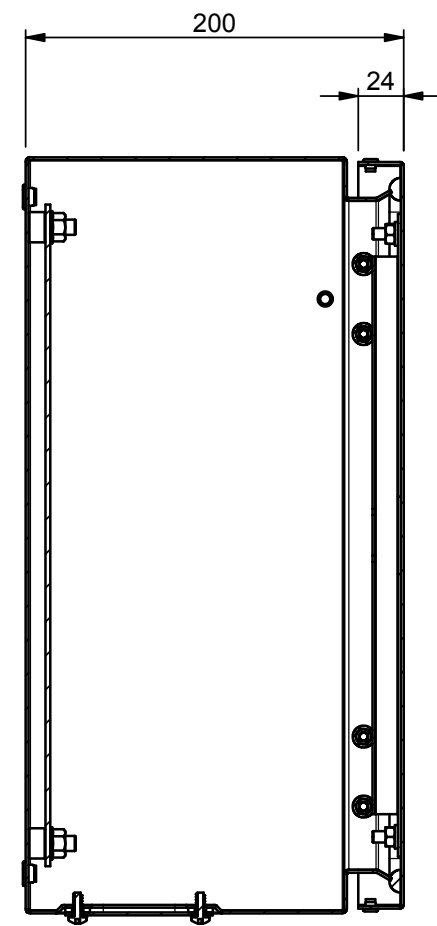
SEZIONE A-A
