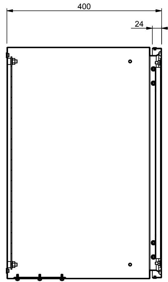
SEZIONE A-A
