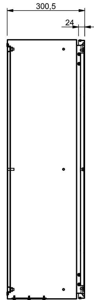
SEZIONE A-A
