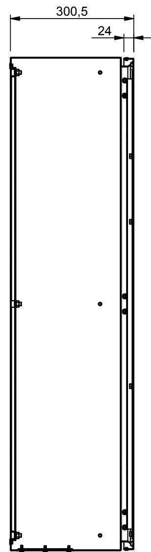
SEZIONE A-A
