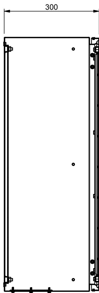
SEZIONE A-A
